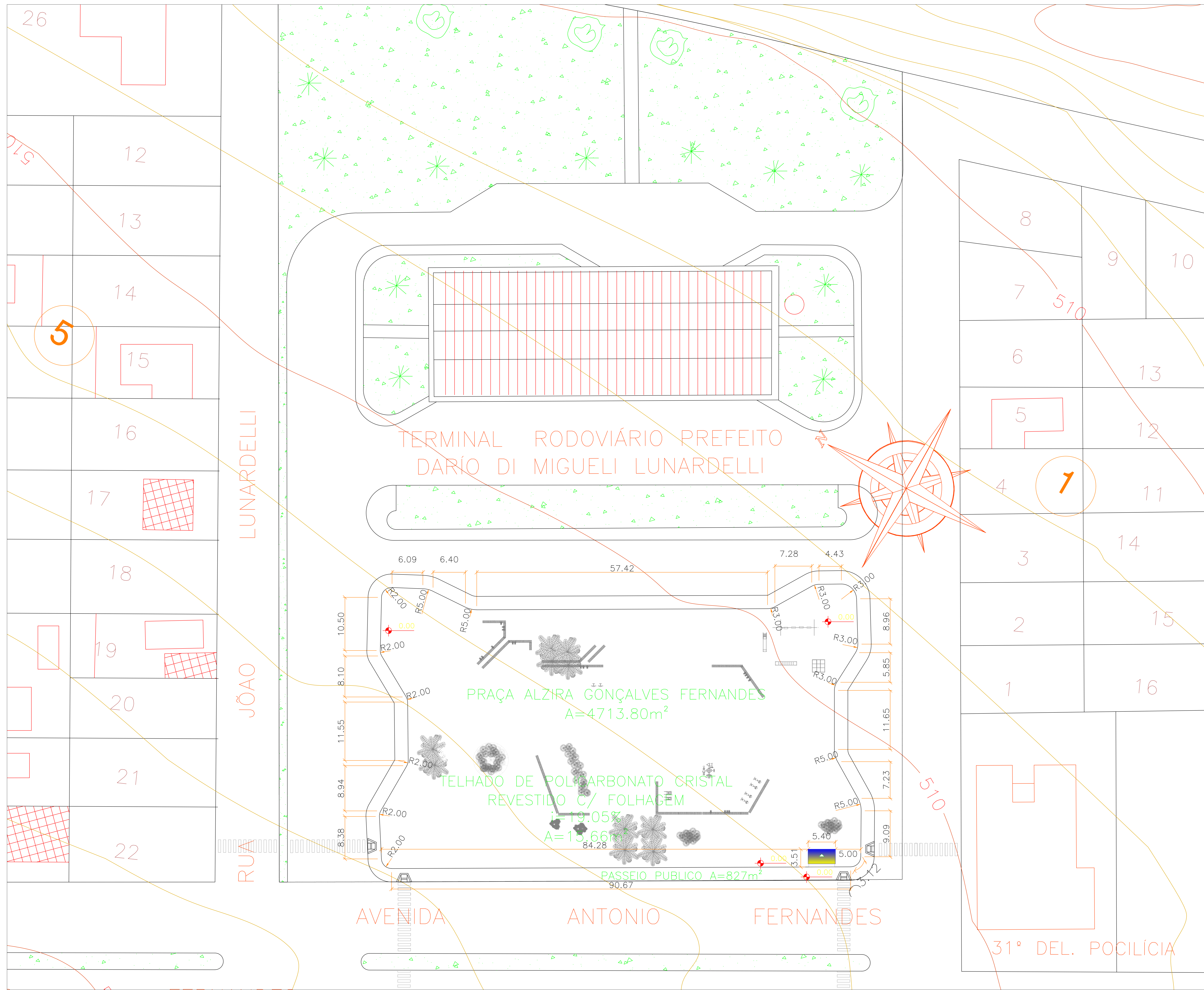
PLANTA IMPLANTAÇÃO esc 1:250
