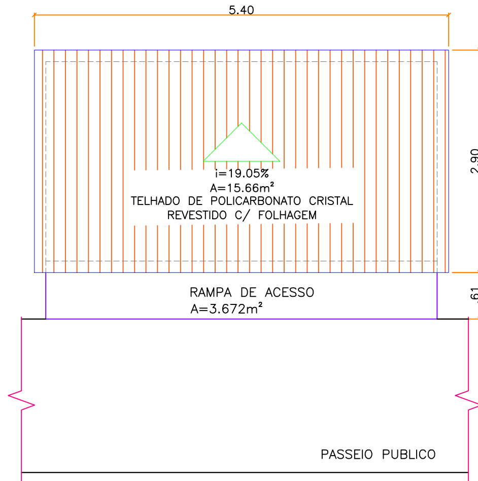
COBERTURA esc 1:50
