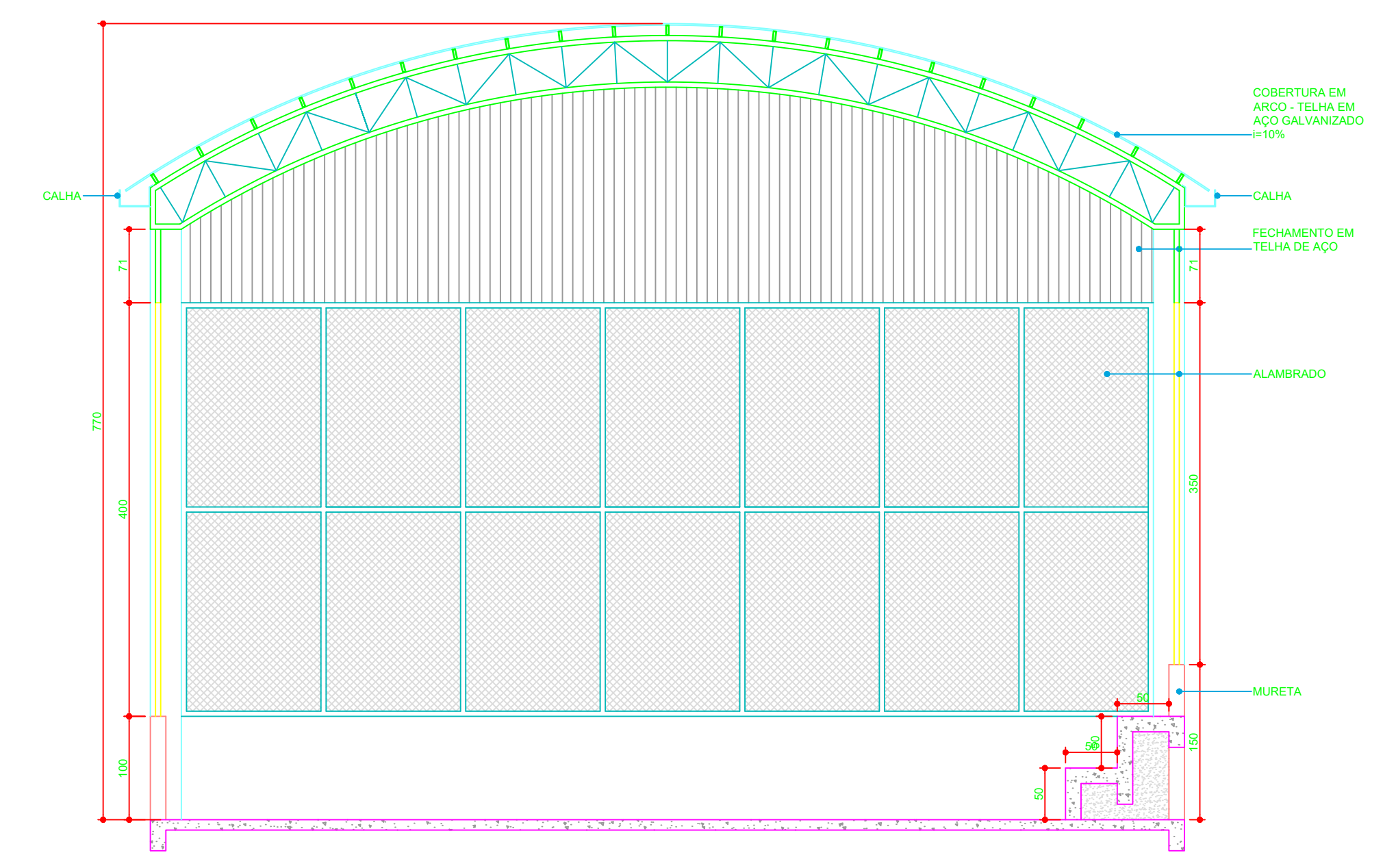
02 1:50 QUADRA POLIESPORTIVA CORTE AA
