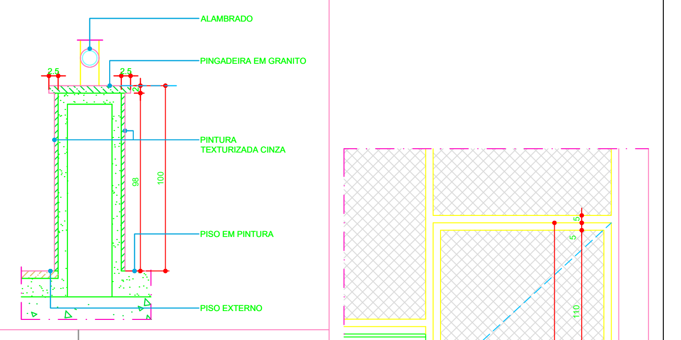
03 1:10 MURETA DETALHE
