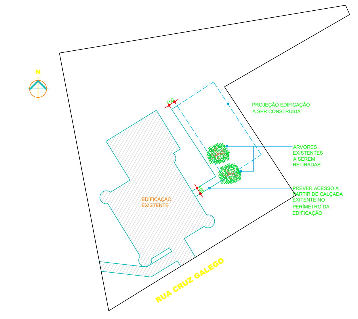
07 1:500 ACESSO E ÁRVORES A SEREM RETIRADAS PLANTA BAIXA
