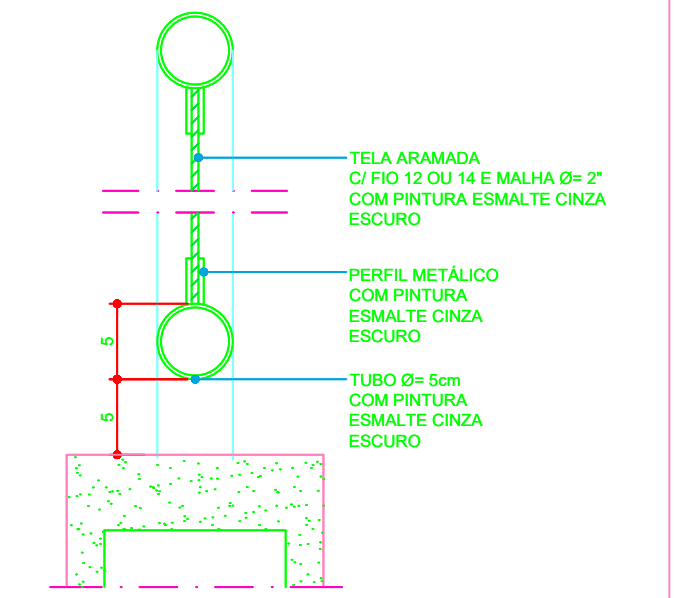
04 1:5 ALAMBRADO DETALHE
